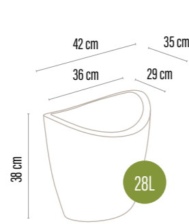
ALYG-13 GONDOL POT NO.1 Gondol Saksı No.1 35 x 42 x 38 cm Ø29 x 36 cm 0,0434 m 3 1450 g
