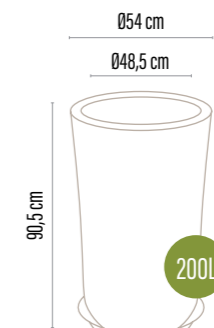
ALYG-20 VİTRİN POT NO.2 Vitrin Saksı No.2 Ø54 x 90,5 cm Ø48,5 cm 0,2638 m 3 5000 g
